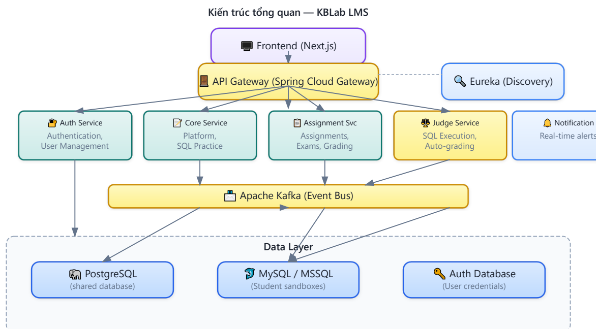
Hình 1.8: Kiến trúc tổng quan hệ thống KBLab LMS
