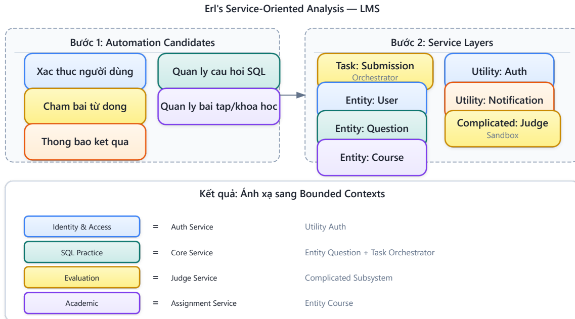
Hình 2.6b: Áp dụng Erl's Service-Oriented Analysis cho LMS — từ automation candidates đến service layers
