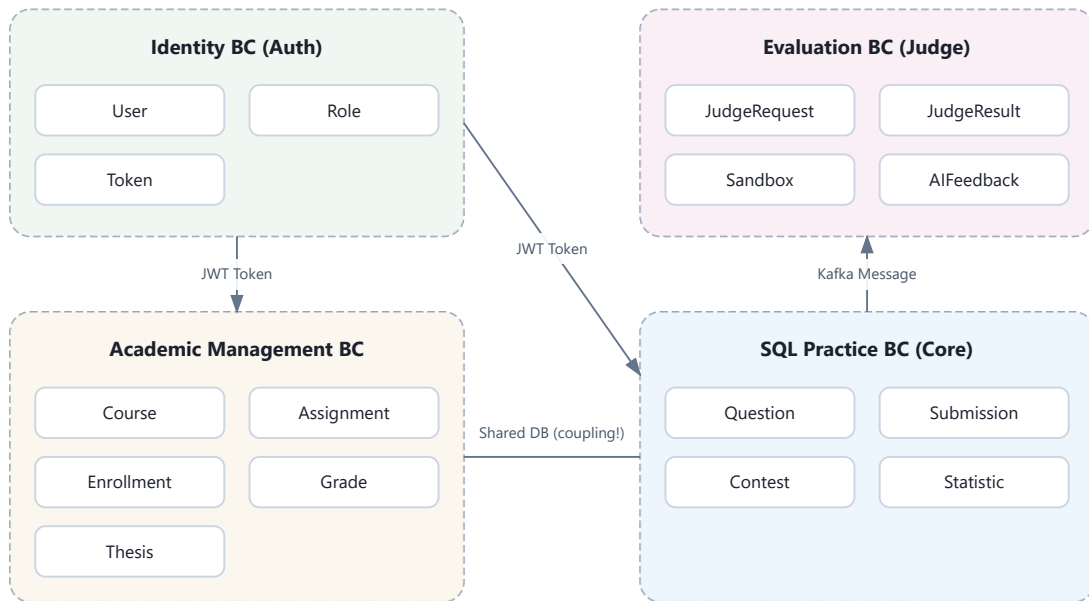
Hình 2.7: Bốn bounded contexts chính trong hệ thống LMS
