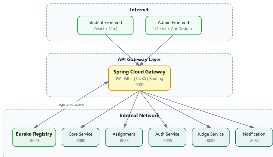
Hình 8.7: Kiến trúc tổng thể LMS — Gateway là single entry point
