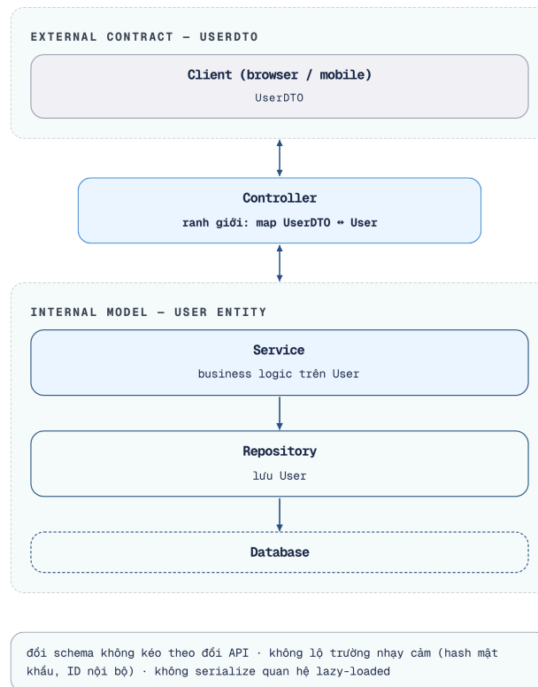
Hình 3.4: DTO pattern — tách internal model và external contract
