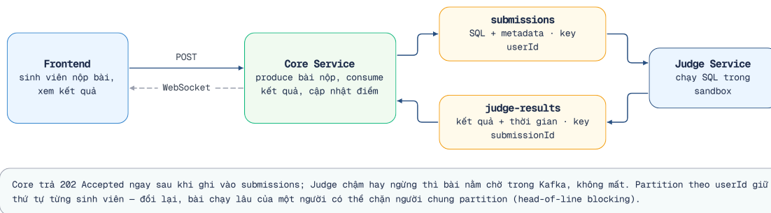
Hình 5.7: Kiến trúc pipeline 2 Kafka topic chấm bài trong chế độ thi
