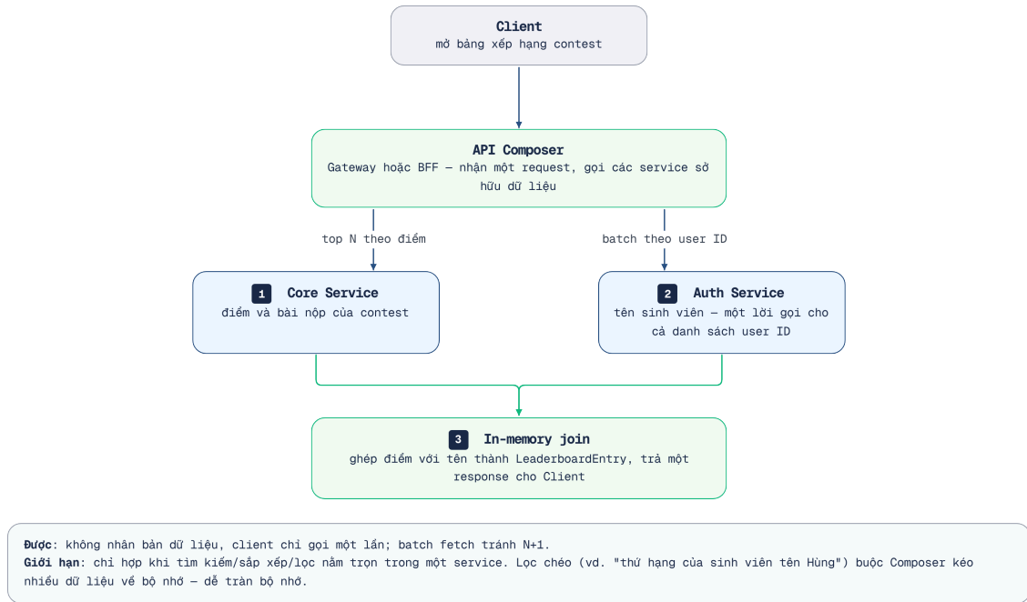
Hình 7.8: API Composition pattern — Gateway hoặc BFF gọi nhiều service rồi tổng hợp
