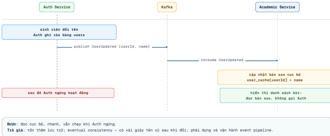
Hình 7.7: Truy cập dữ liệu xuyên service bằng Data Duplication qua Event Pipeline
