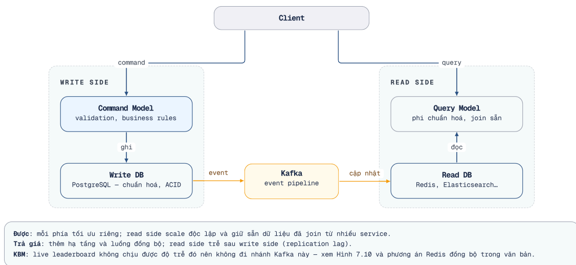
Hình 7.9: CQRS pattern — tách command model (write) và query model (read)
