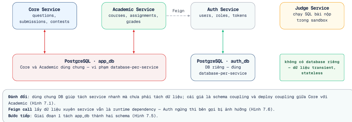
Hình 7.14: Kiến trúc dữ liệu hiện tại của KBM – shared database là thiếu sót chính
