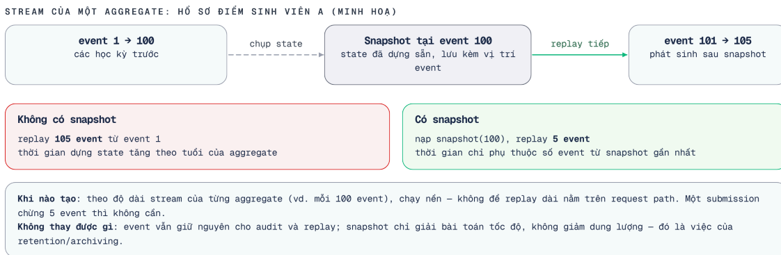
Hình 7.12: Snapshot pattern — replay từ snapshot thay vì từ đầu
