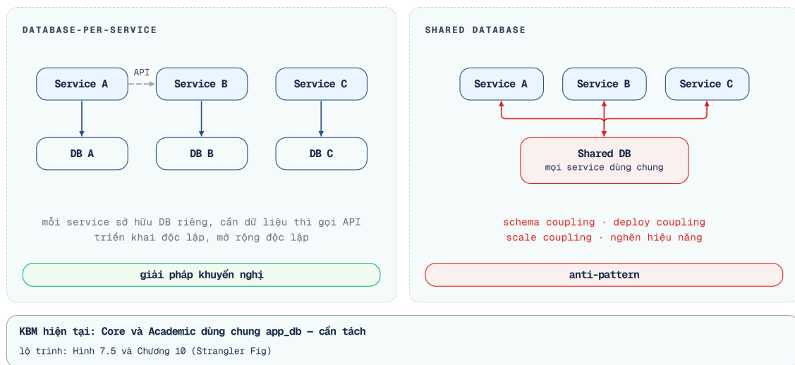
Hình 7.2: Shared Database (đọc/ghi chung) vs Database-per-Service (dữ liệu qua API)
