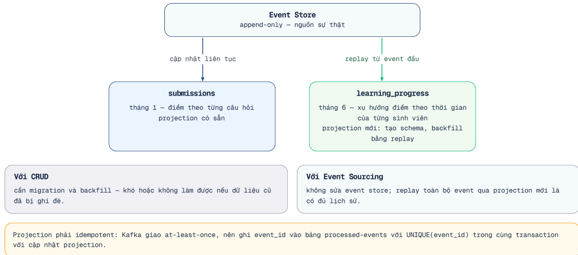
Hình 7.13: Projection Rebuilds — tạo view mới từ event mà không cần migration schema
