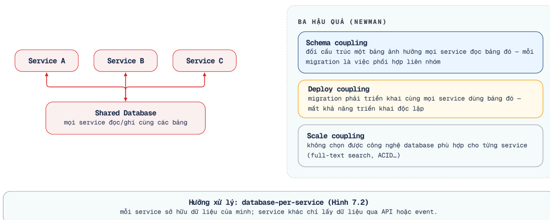
Hình 7.1: Ba hậu quả của shared database trong microservices
