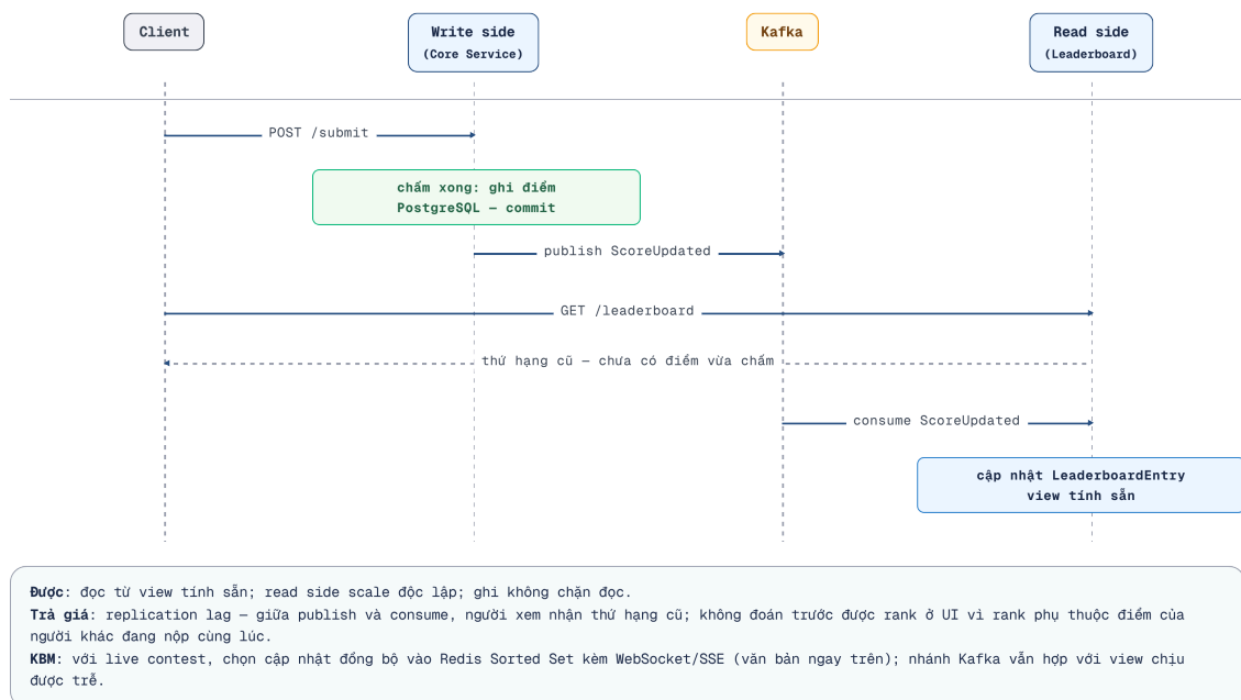
Hình 7.10: Đường CQRS bất đồng bộ qua Kafka cho Leaderboard — luồng này sinh replication lag; phương án đồng bộ Redis Sorted Set được mô tả trong văn bản
