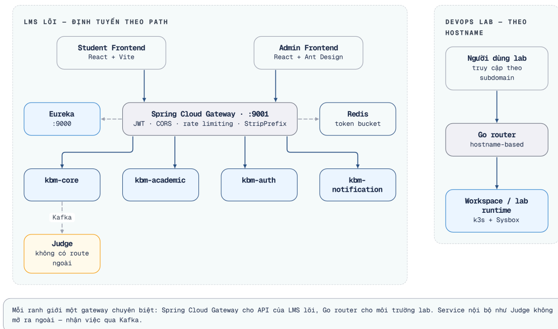
Hình 8.7: Kiến trúc tổng thể KBM — Gateway là single entry point
