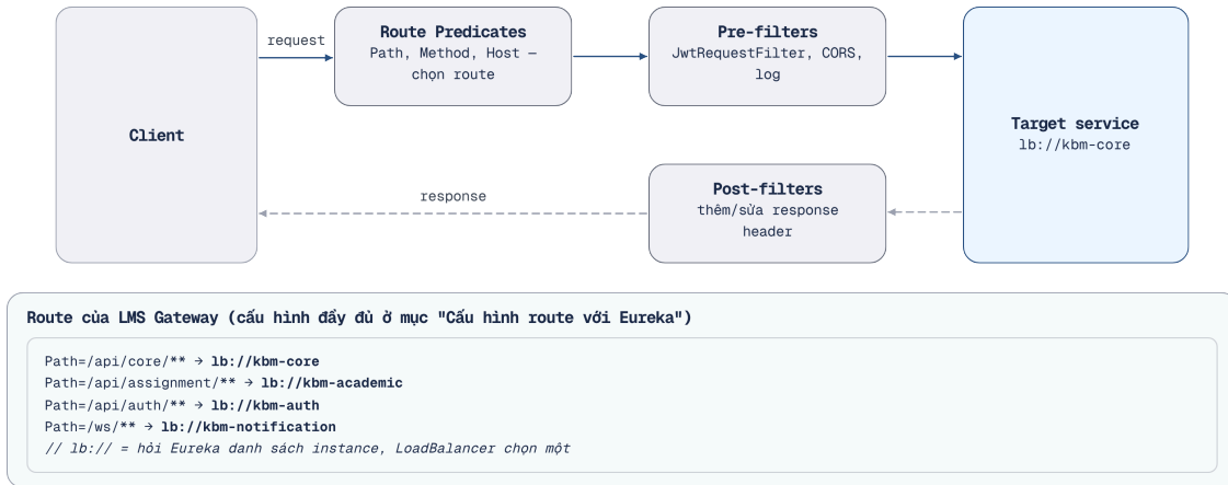
Hình 8.4: Kiến trúc Spring Cloud Gateway — Predicates, Filters, Routes
