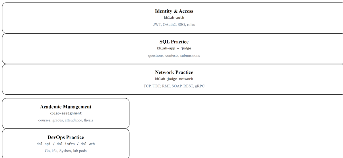
Hình 2.7: Năm bounded contexts chính trong KBLab
