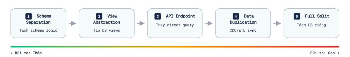
Hình 10.4: Thứ tự thực hiện 5 chiến lược tách database
