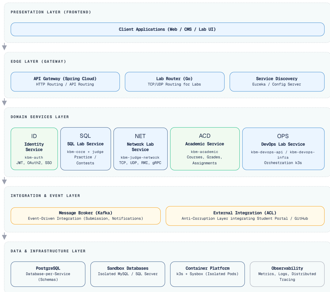
Hình 1.8: Kiến trúc tổng quan hệ thống KBM LMS (sơ đồ giản lược theo năm context ban đầu — bức tranh đầy đủ 7 core + 2 supporting bounded context được trình bày ở Chương 2)
