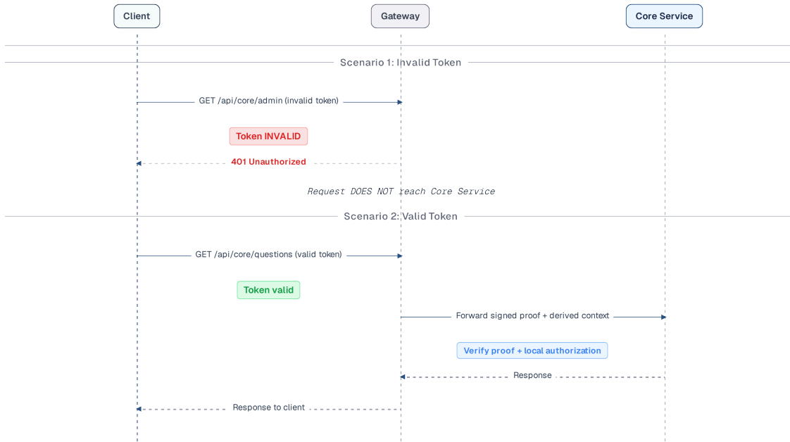
Hình 8.6: Luồng JWT tại Gateway — bằng chứng có chữ ký và context định danh dẫn xuất
