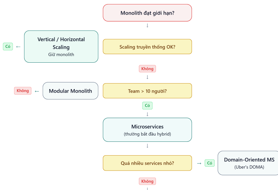
Hình 1.4: Cây quyết định chuyển đổi kiến trúc — từ monolith đến microservices
