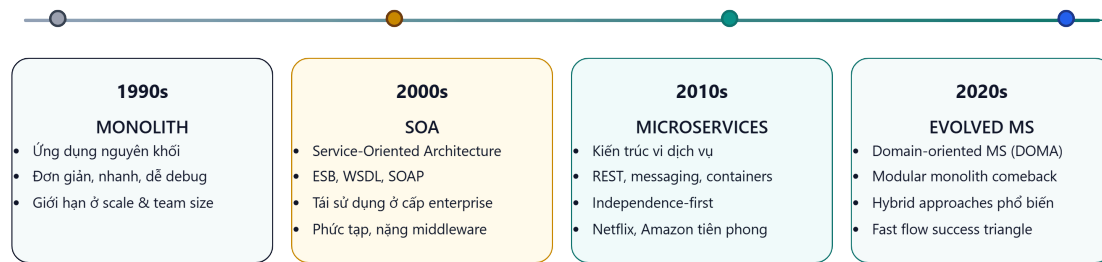
Hình 1.1: Tiến hóa kiến trúc phần mềm doanh nghiệp từ thập niên 1990 đến 2020
