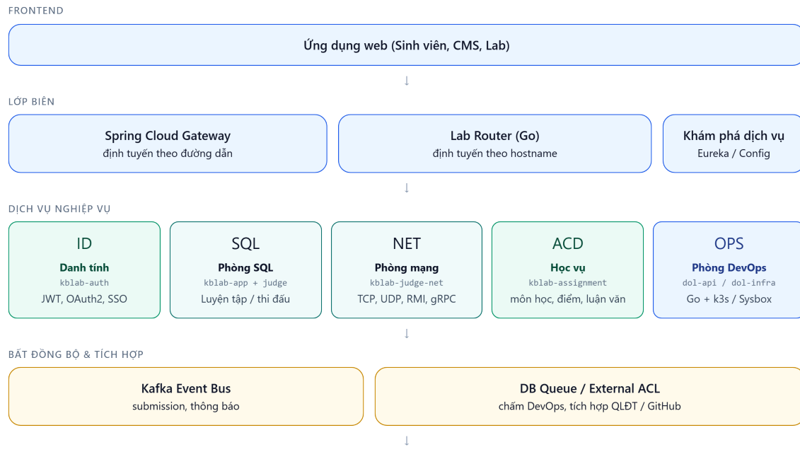
Hình 1.8: Kiến trúc tổng quan hệ thống KBLab LMS
