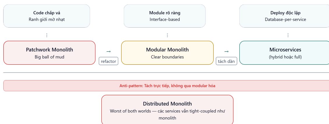
Hình 1.6: Con đường từ Patchwork Monolith đến Microservices
