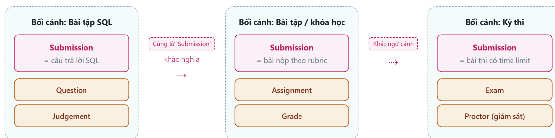
Hình 2.4: Cùng thuật ngữ “Submission” mang ý nghĩa khác nhau trong ba bounded context
