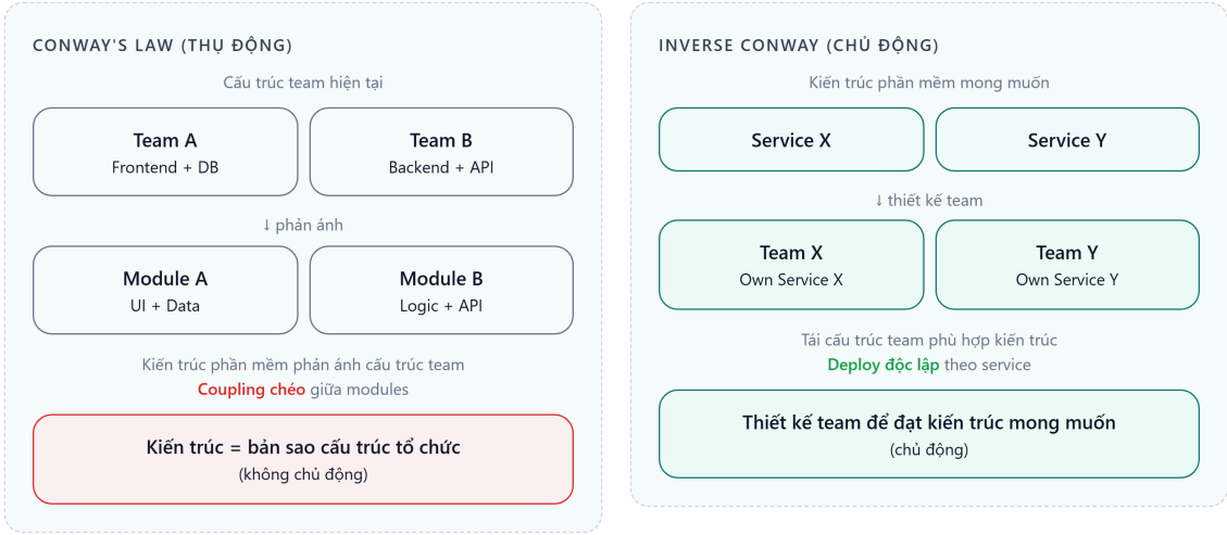
Hình 2.1: Conway’s Law (thụ động) vs Inverse Conway Maneuver (chủ động)
