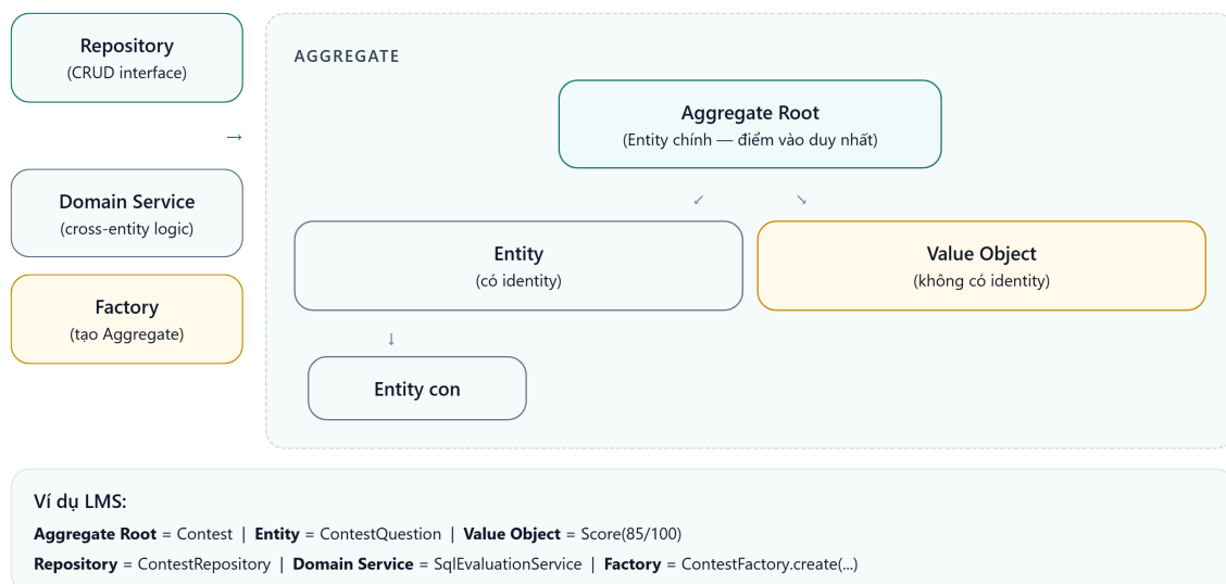
Hình 2.3: Các building blocks trong DDD — Aggregate, Entity, Value Object, Repository
