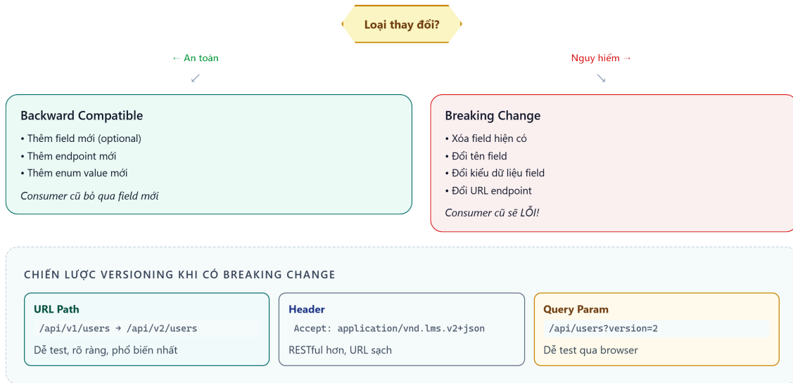
Hình 3.2: Quy tắc schema evolution — thay đổi nào là breaking change
