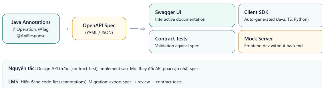
Hình 3.3: Pipeline từ code annotations đến Swagger UI và client SDK
