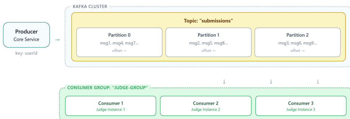
Hình 5.5: Kiến trúc Kafka — Topic, Partitions và Consumer Group
