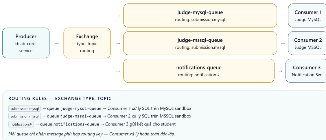
Hình 5.4: Kiến trúc RabbitMQ — Exchange routing messages đến queues
