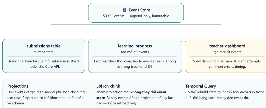
Hình 7.13: Projection Rebuilds — tạo views mới từ events mà không cần migration
