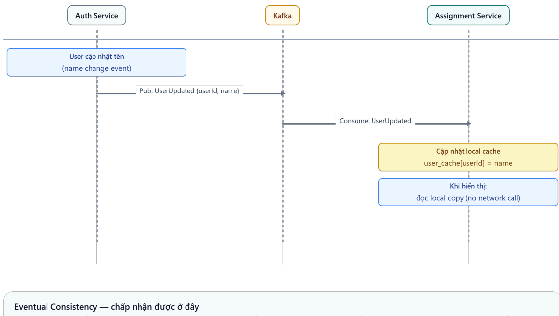
Hình 7.8: Truy cập dữ liệu xuyên service bằng Data Duplication qua Event Pipeline
