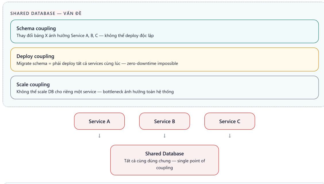
Hình 7.1: Ba hậu quả của shared database trong microservices
