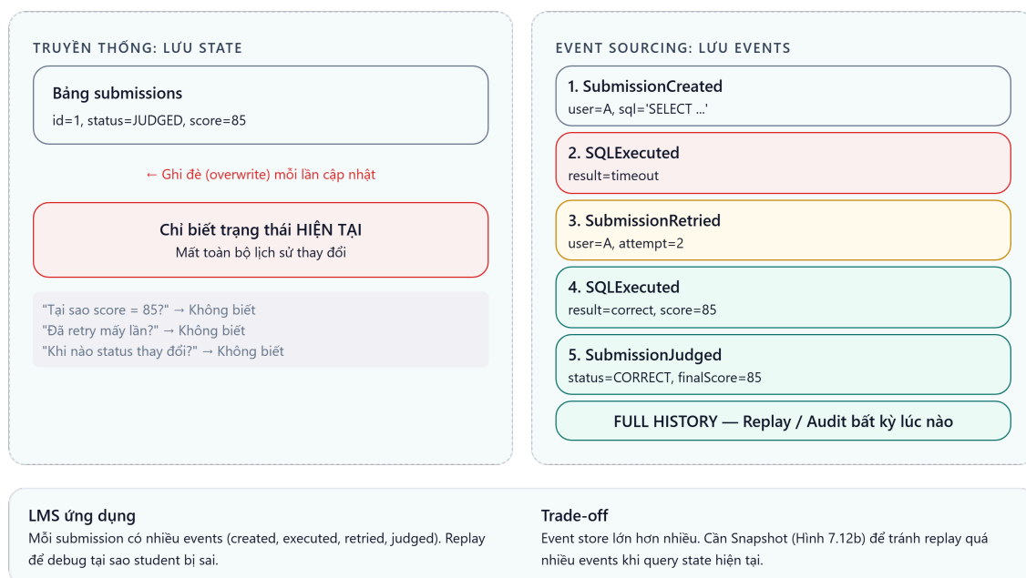
Hình 7.12: Event Sourcing — lưu chuỗi events thay vì chỉ state hiện tại
