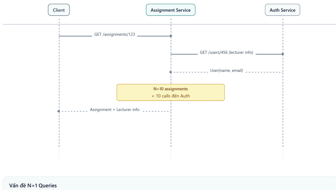
Hình 7.7: Truy cập dữ liệu xuyên service bằng API Call
