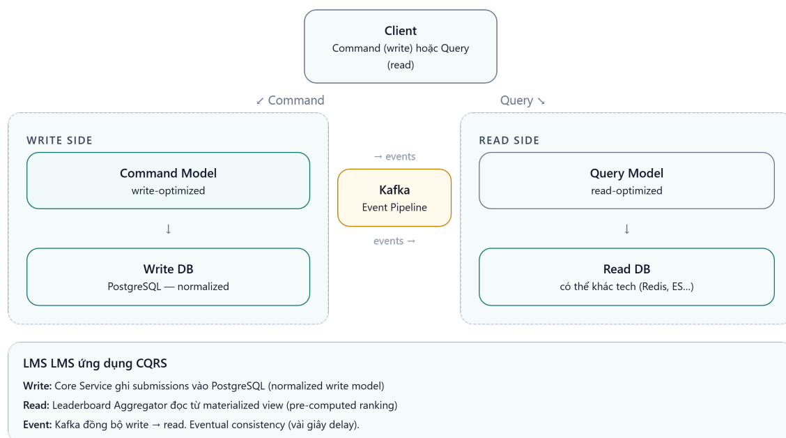
Hình 7.10: CQRS pattern — tách command model (write) và query model (read)
