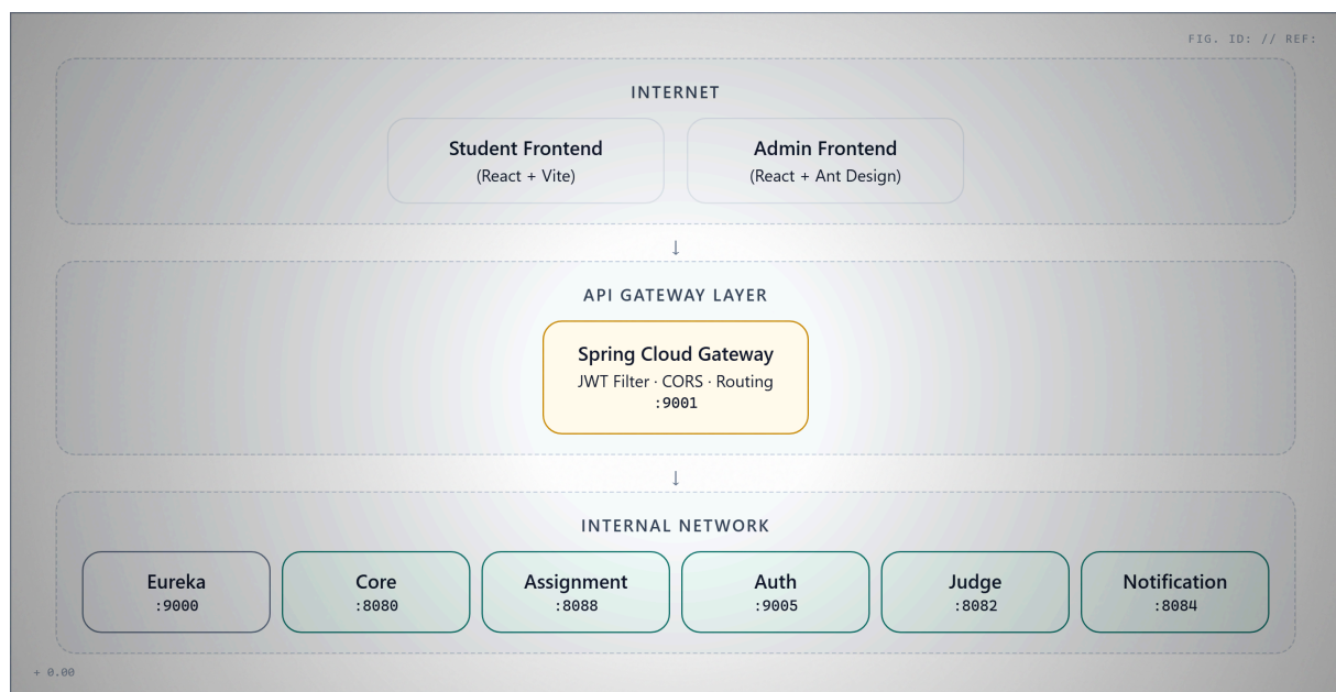
Hình 8.7: Kiến trúc tổng thể KBLab — Gateway là single entry point
