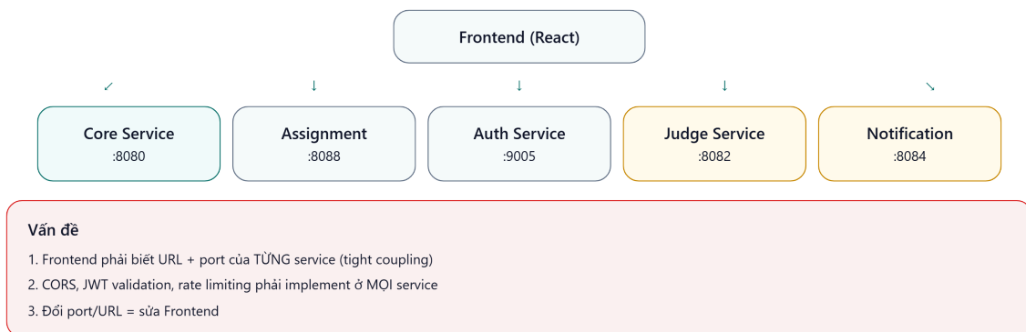
Hình 8.1: Không có Gateway — client phải biết địa chỉ của từng service
