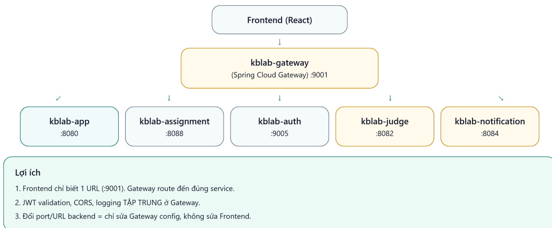
Hình 8.2: API Gateway — single entry point route đến từng service
