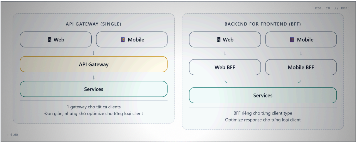
Hình 8.3: API Gateway (một gateway chung) vs BFF (gateway riêng cho từng client)
