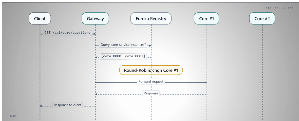
Hình 8.5: Luồng lb:// — Eureka lookup + load balance + route
