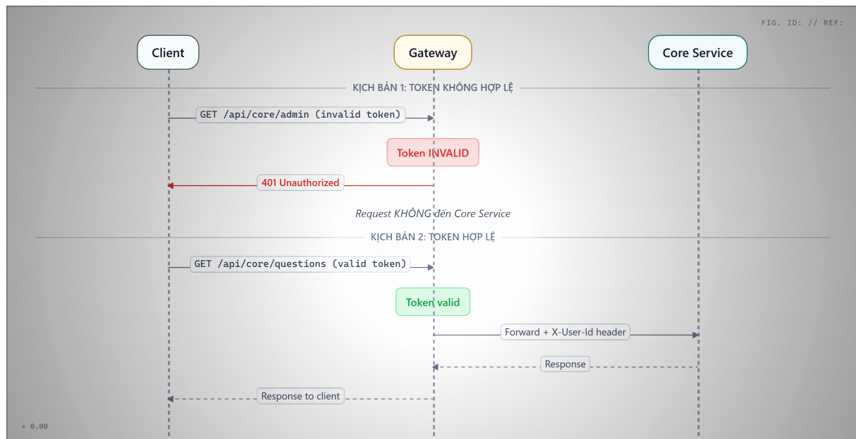
Hình 8.6: Luồng JWT validation tại Gateway — claims propagation qua trusted headers
