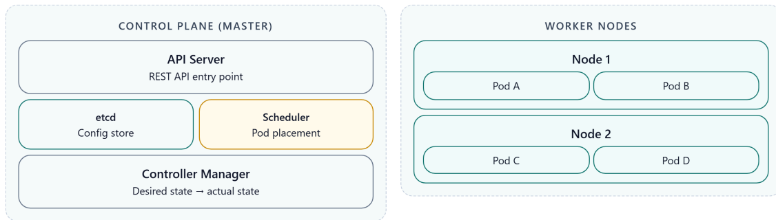
Hình 12.6: Kiến trúc Kubernetes — Control Plane và Worker Nodes
