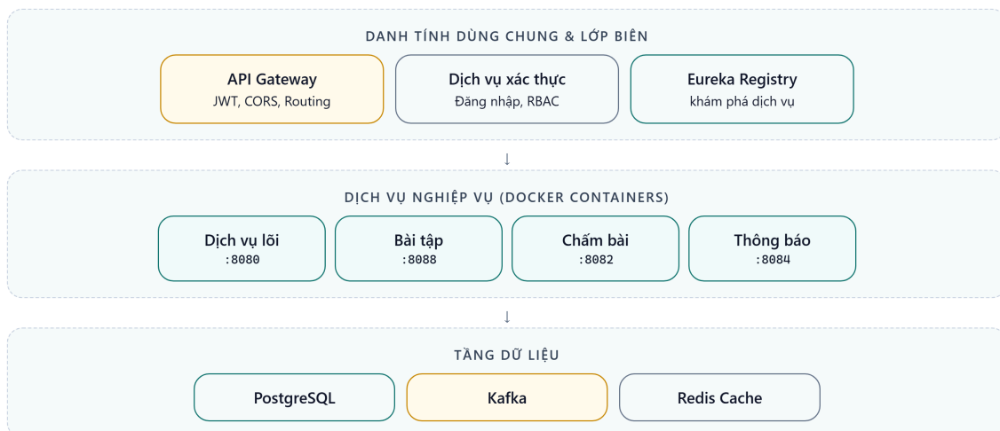
Hình 12.8: Deployment Architecture KBLab ở mức khái quát
