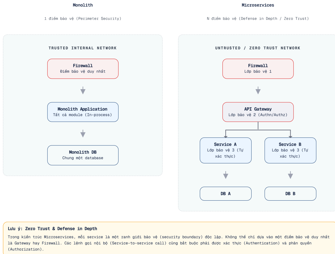
Hình 9.1: Monolith (1 điểm bảo vệ) vs Microservices (N điểm bảo vệ)
