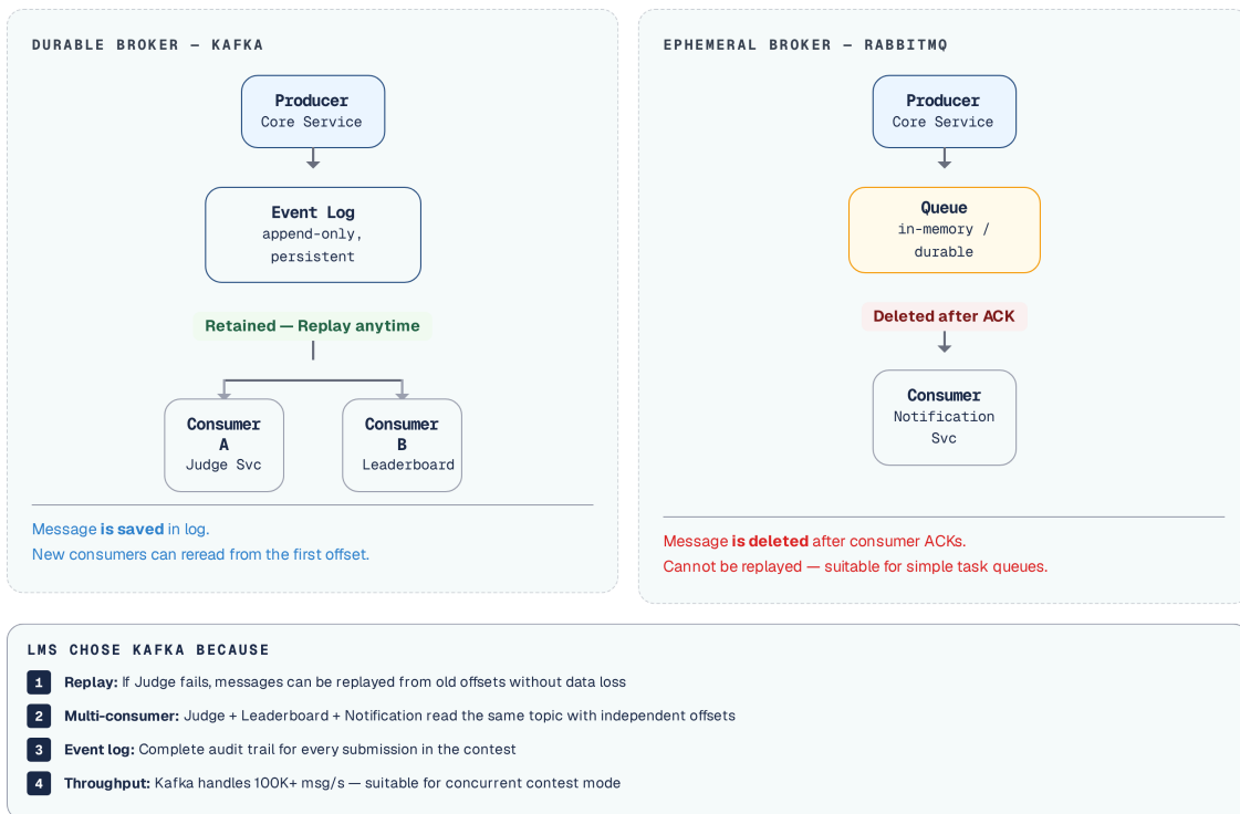
Hình 5.3: Ephemeral broker (message xóa sau ack) vs Durable broker (message vẫn còn)
