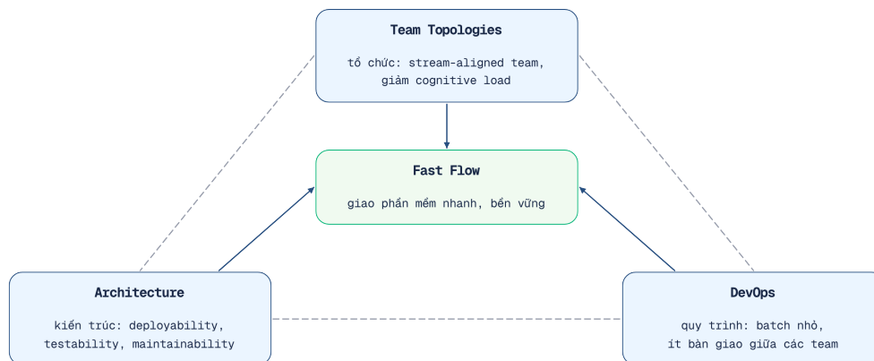
Hình 1.5: Fast Flow Success Triangle — ba yếu tố cần thiết cho fast flow
