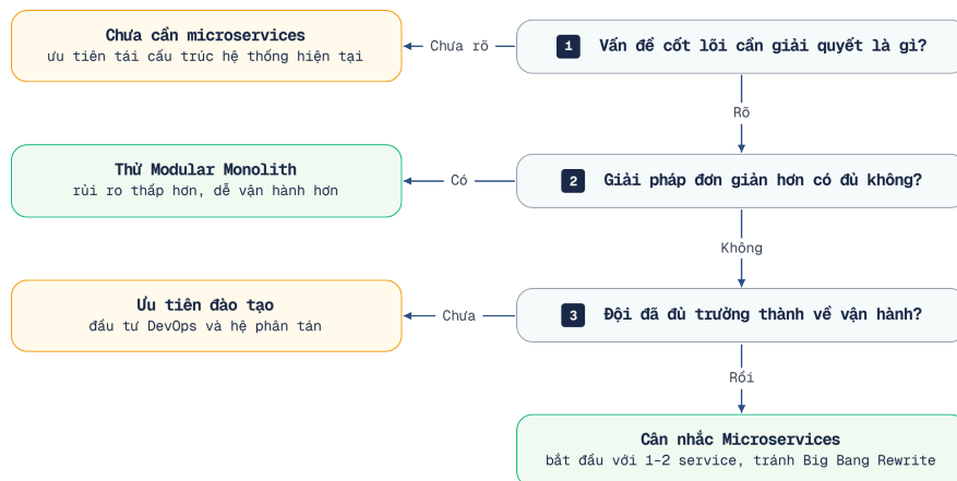
Hình 1.7: Khung ra quyết định (Decision Framework) — ba câu hỏi trước khi chọn microservices
