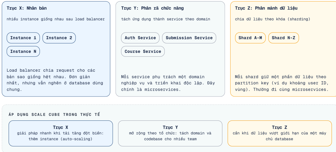
Hình 1.3: Scale Cube — ba chiều mở rộng hệ thống
