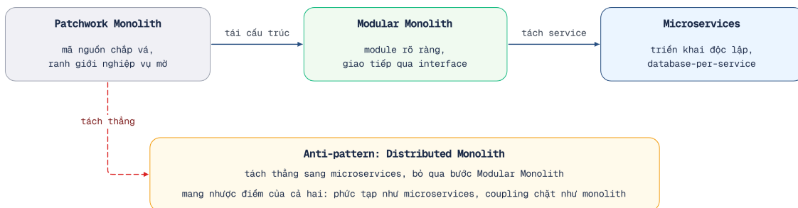
Hình 1.6: Con đường từ Patchwork Monolith đến Microservices
