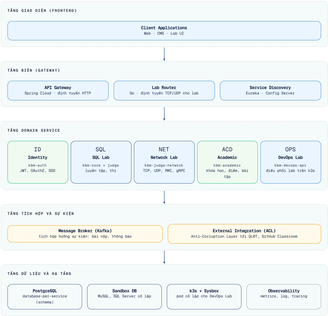
Hình 1.8: Kiến trúc tổng quan hệ thống KBM LMS (sơ đồ giản lược theo năm context ban đầu — bức tranh đầy đủ 7 core + 2 supporting bounded context được trình bày ở Chương 2)
