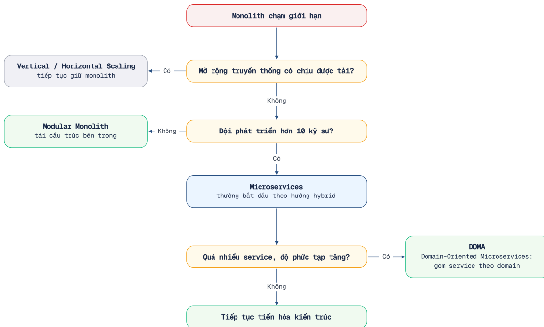
Hình 1.4: Cây quyết định chuyển đổi kiến trúc — từ monolith đến microservices
