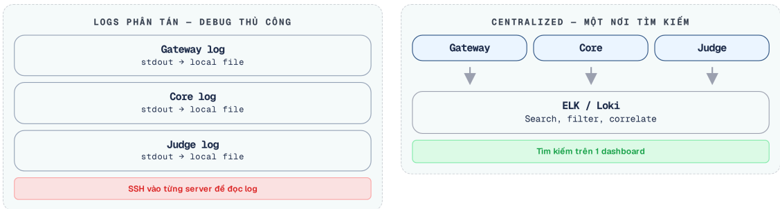
Hình 11.3: Logs phân tán (manual debug) vs Logs tập trung — Search một nơi
