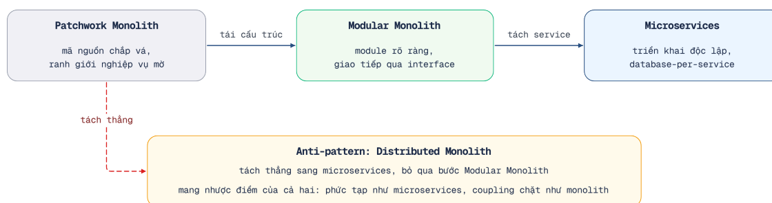
Hình 1.6: Con đường từ Patchwork Monolith đến Microservices
