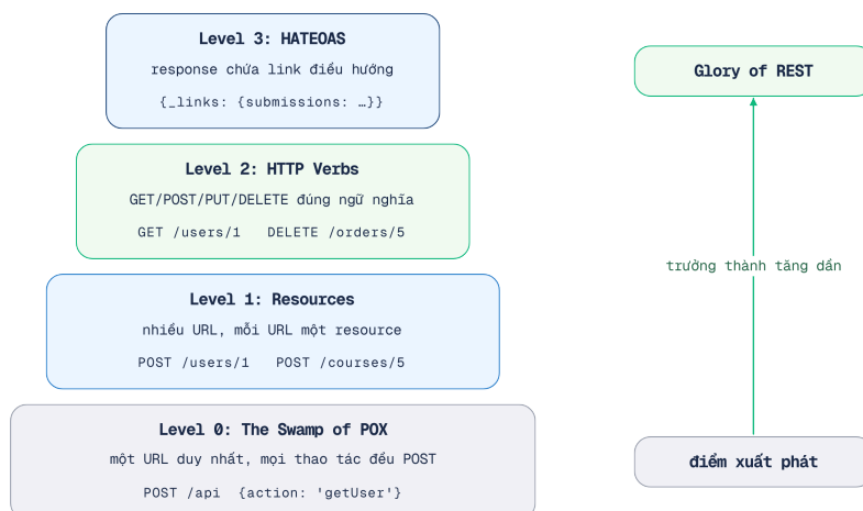
Hình 3.1: Richardson Maturity Model — bốn cấp độ trưởng thành của REST API
