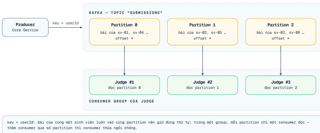
Hình 5.5: Kiến trúc Kafka — Topic, Partitions và Consumer Group
