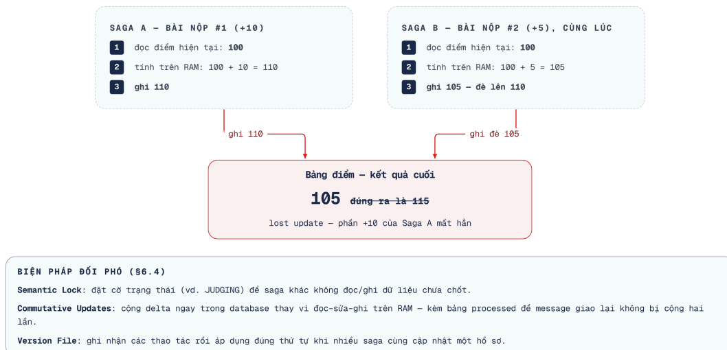
Hình 6.5: Lost Updates anomaly — hai saga ghi đè kết quả của nhau
