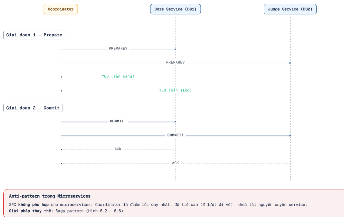
Hình 6.1: Two-Phase Commit — Coordinator điều phối prepare và commit
