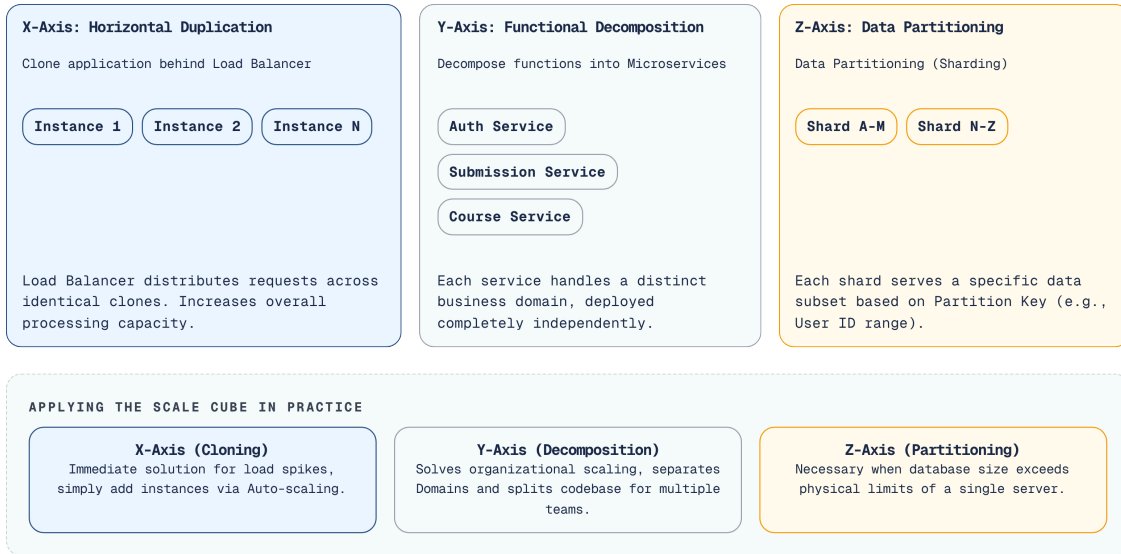
Hình 1.3: Scale Cube — ba chiều mở rộng hệ thống
