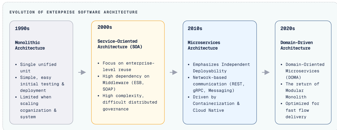
Hình 1.1: Tiến hóa kiến trúc phần mềm doanh nghiệp từ thập niên 1990 đến 2020
