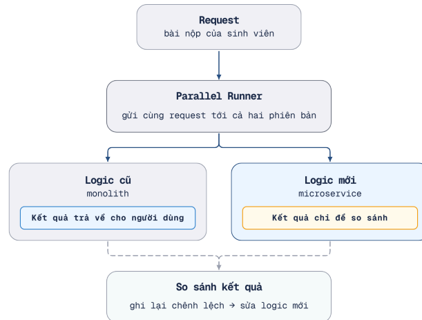
Hình 10.9: Parallel Run — chạy song song logic cũ và mới, so sánh kết quả
