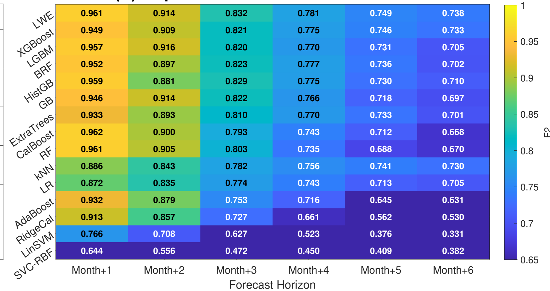
(D) Model comparison — All datasets
