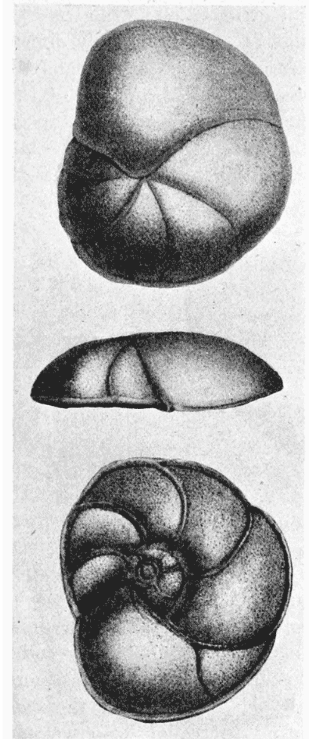
Fig. 316. Discorbina berthelotti , d'Orb.
