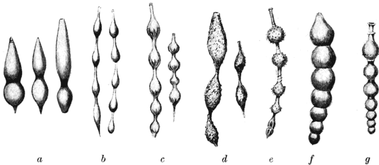
Fig. 89. Various Foraminifera (after Brady), a , Nodosaria simplex ; b , N. pygmaea ; c , N. costulata ; e , N. hispida ; f , N. elata ; d , Rheophax ( Lituola ) distans ; g , Sagrina virgata .
