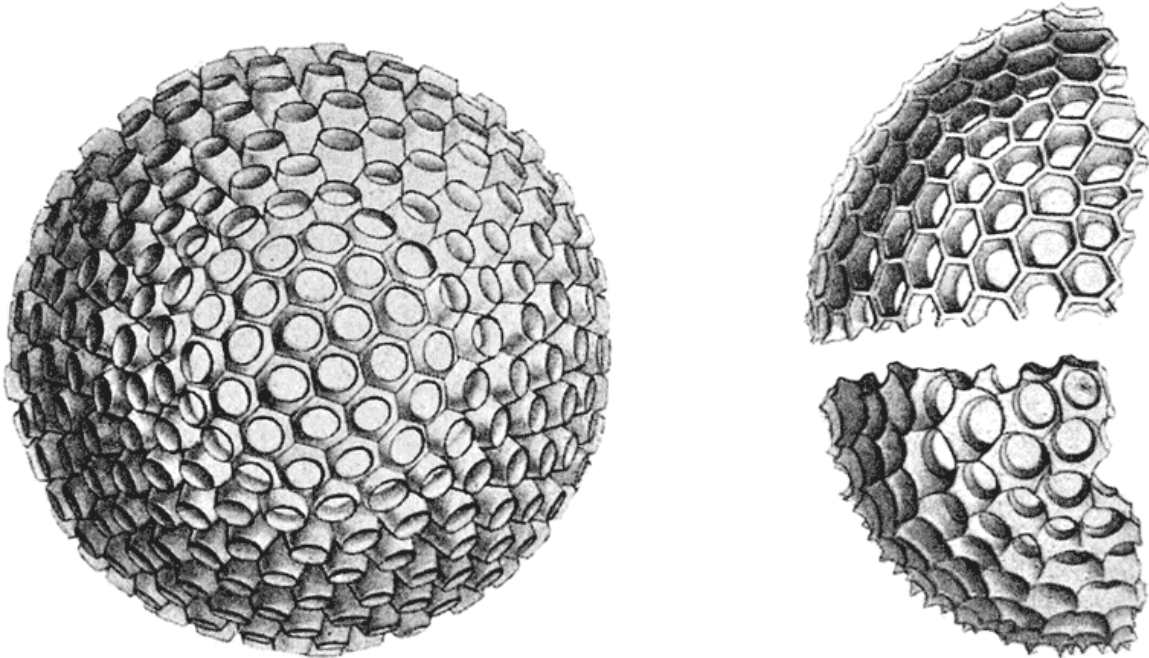
Fig. 223. Ethmosphaera conosiphonia , Hkl.
