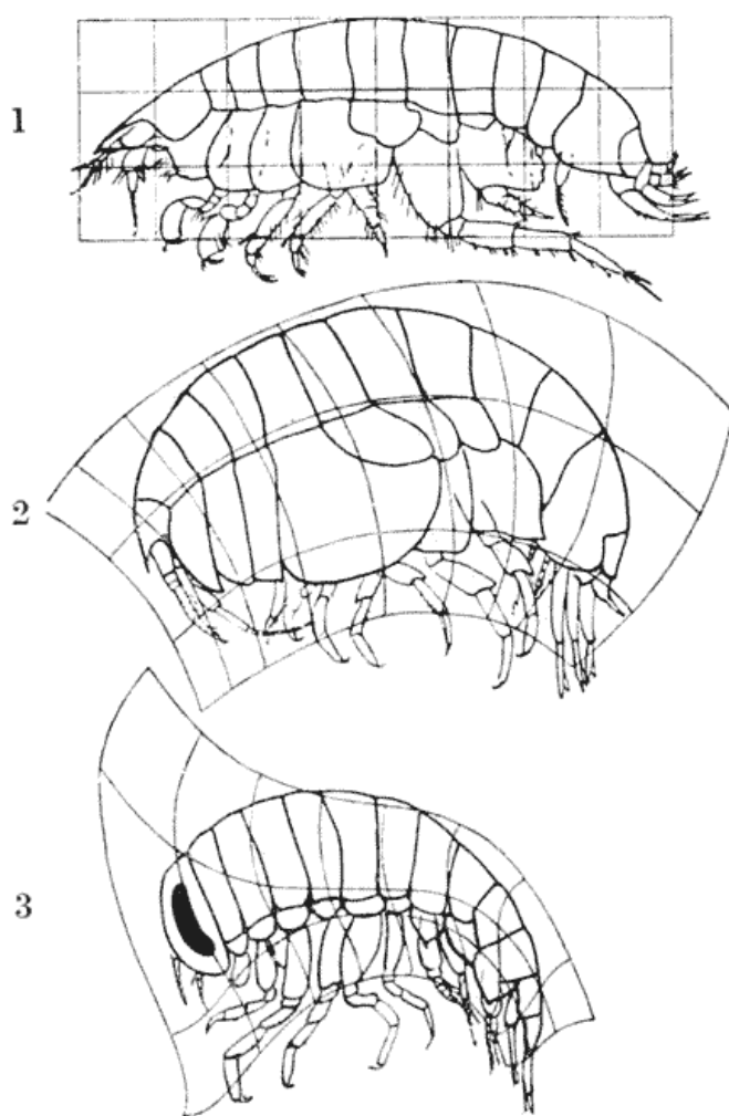
Fig 370. 1. Harpinia plumosa Kr. 2. Stegocephalus inflatus Kr. 3. Hyperia galba .
