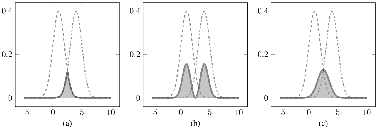
Hình 1.3. Minh họa khoảng cách \mathcal{L}_2 và một vài Affinity phổ biến giữa hai hàm mật độ Gauss \mathcal{N}(1, 1) và \mathcal{N}(4, 1)
