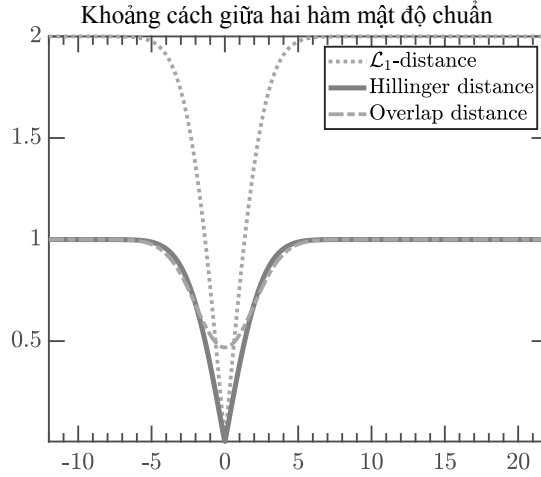
Hình 1.4. Dãy khoảng cách giữa hai hàm mật độ Gauss \mathcal{N}(0, 1) và \mathcal{N}(\mu, 1)
