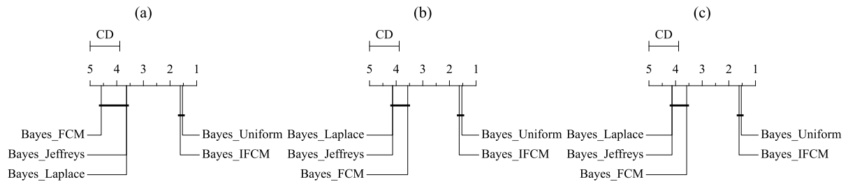
Hình 2.12. Kết quả ANOVA cho các chỉ số phân loại đối với Ví dụ 2.2 Chú thích: (a) Độ chính xác ACC, (b) Độ chính xác cân bằng GM và (c) Chỉ số F_1 -score.
