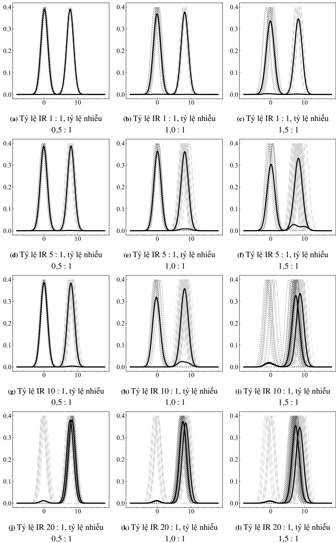
Hình 2.2. Ảnh hưởng của dữ liệu hàm mật độ Gauss mất cân bằng lên FCF ( m = 2; c = 3; D = \mathcal{L}_2 )
