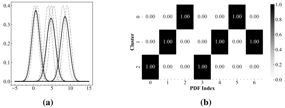
Hình 1.5: Kết quả trọng tâm và ma trận phân vùng của thuật toán KCF đối với Ví dụ 1.4 Chú thích: Hình (a) PDF trọng tâm cụm bằng nét liền và dữ liệu PDF nét đứt ở các cụm, và (b) ma trận phân vùng cứng của KCF. Nguồn: Minh họa của tác giả.
