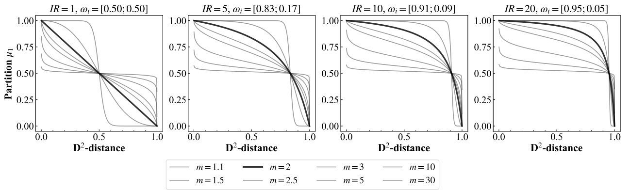
Hình 2.2. Ảnh hưởng của tham số mờ m trong EM-IFCM qua IR
