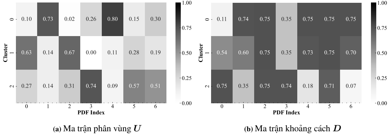
Hình 3.3. Khởi tạo ngẫu nhiên của FCF
