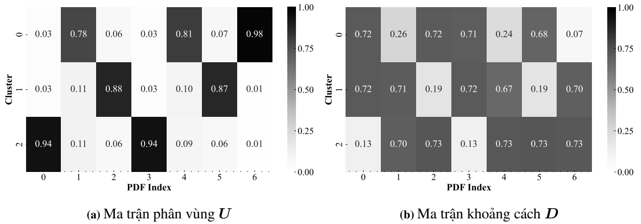
Hình 3.5. Vòng lặp t = 9 của FCF
