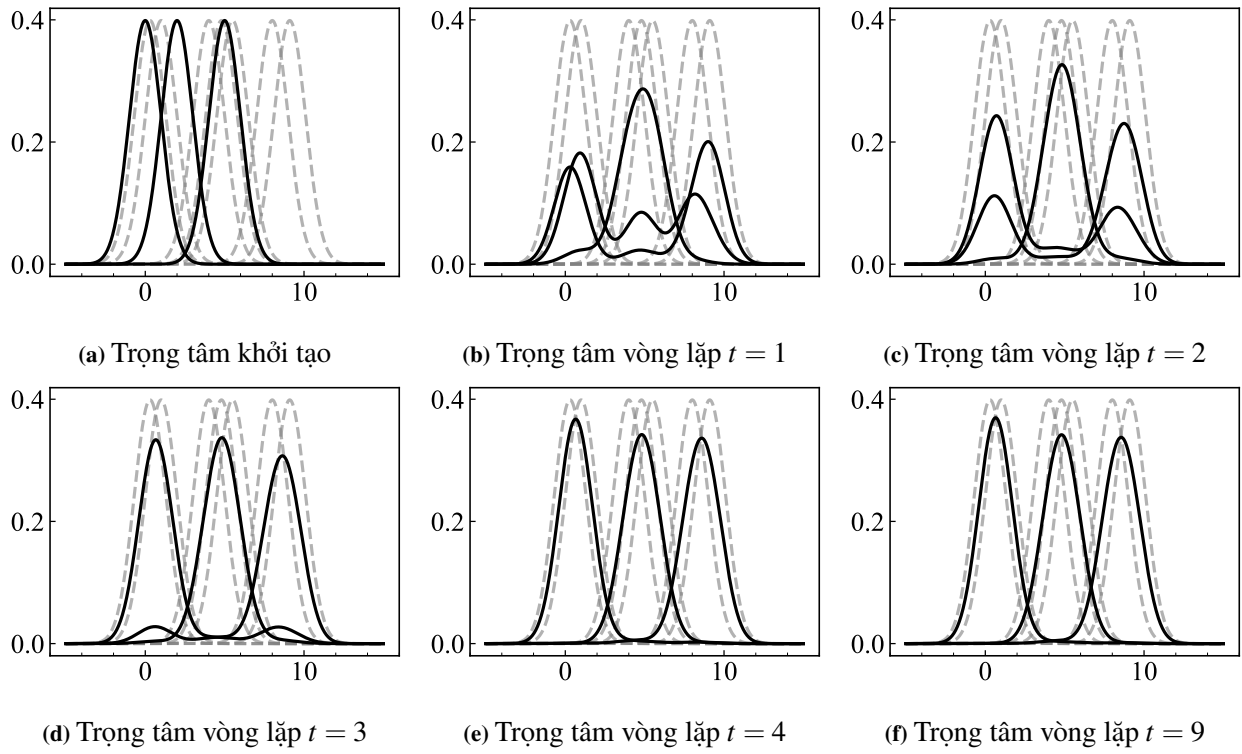
Hình 3.6. Thay đổi của trọng tâm chùm FCF qua các vòng lặp
