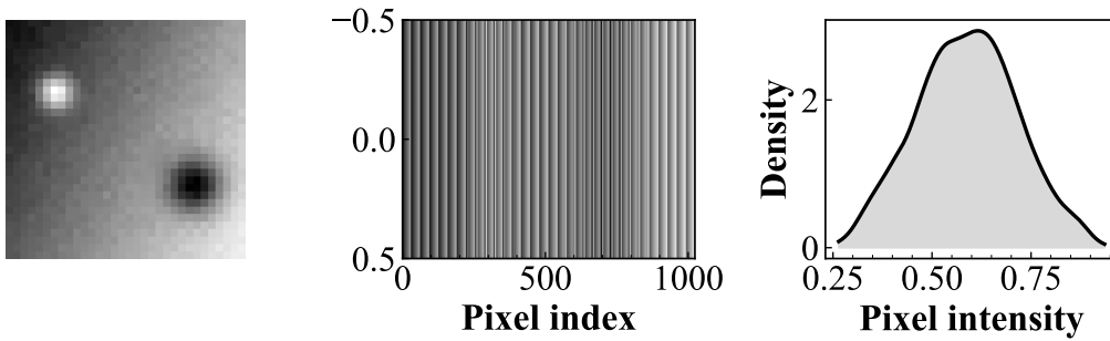
Hình 3.1. Minh họa quá trình chuyển đổi dữ liệu ảnh thành hàm mật độ.
