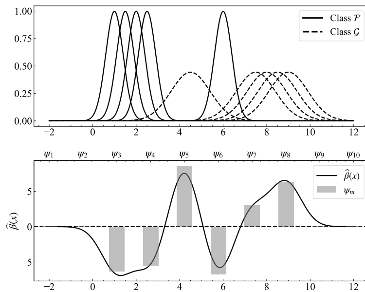
Hình 1.8: Hàm \hat{\beta}(x) được ước lượng qua 10 hàm cơ sở Gauss.
