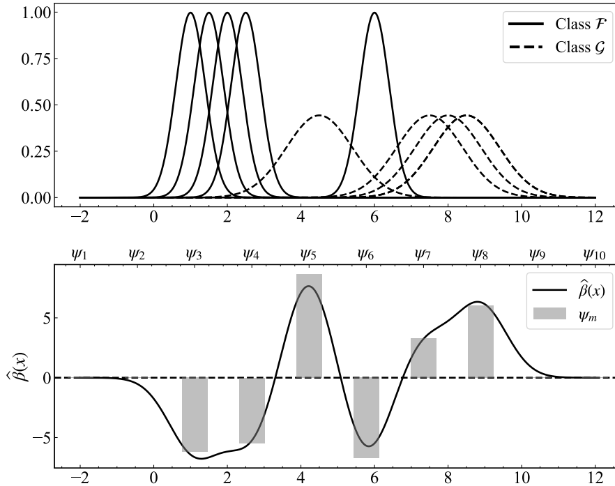
Hình 1.7. Hàm \hat{\beta}(x) được ước lượng qua 10 hàm cơ sở Gauss.
