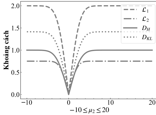
Hình 1.3. Dãy khoảng cách D(f_1, f_2) giữa hai hàm mật độ Gauss \mathcal{N}(0, 1) và \mathcal{N}(\mu, 1)
