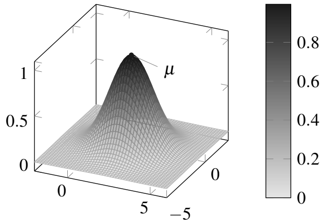
(b) Hàm mật độ Gauss hai chiều
