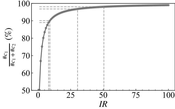
Hình 2.2: Quan hệ giữa tỷ lệ mất cân bằng và quy mô chùm có số lượng chiếm ưu thế
