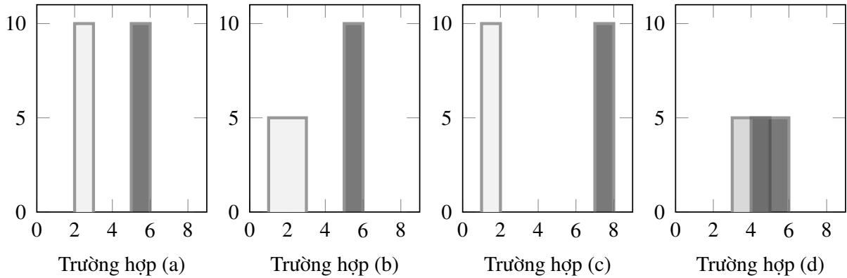
Hình 1.4: Các trường hợp trong khoảng cách giữa hai hàm mật độ đều f_1(x) và f_2(x) đối với Ví dụ 1.1.
