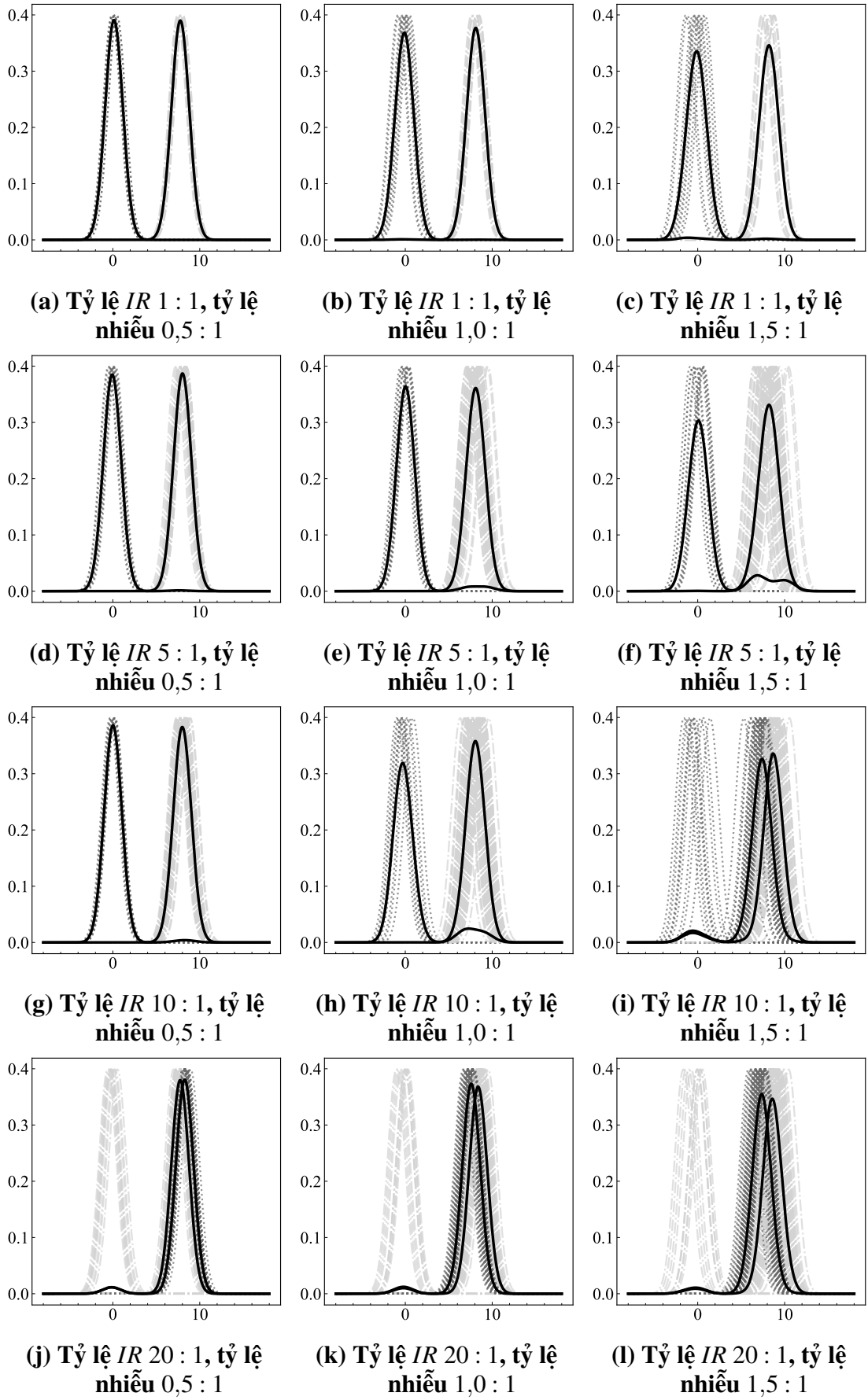
Hình 2.3: Ảnh hưởng của dữ liệu PDF Gauss mất cân bằng lên FCF (m = 2; c = 2; D = \mathcal{L}_2^2)
