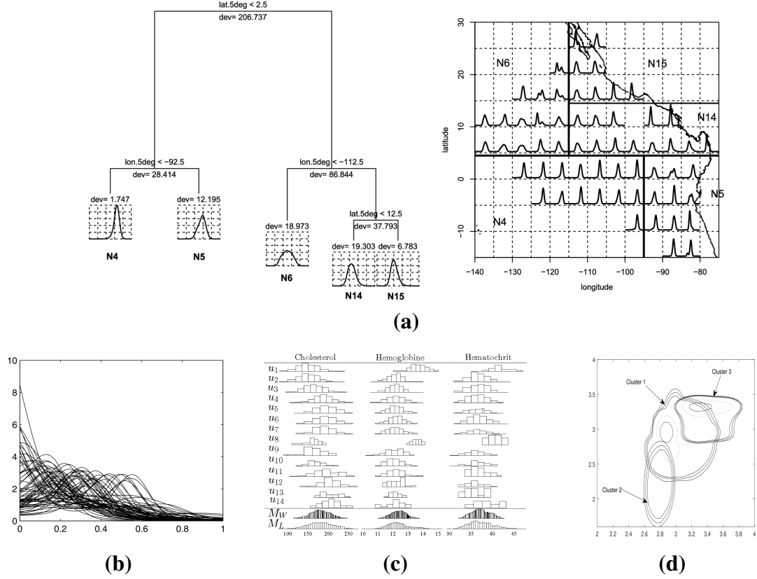
Hình 2.1: Minh họa các dữ liệu hàm mật độ được thu thập trong thực tế từ các nghiên cứu trước đây
