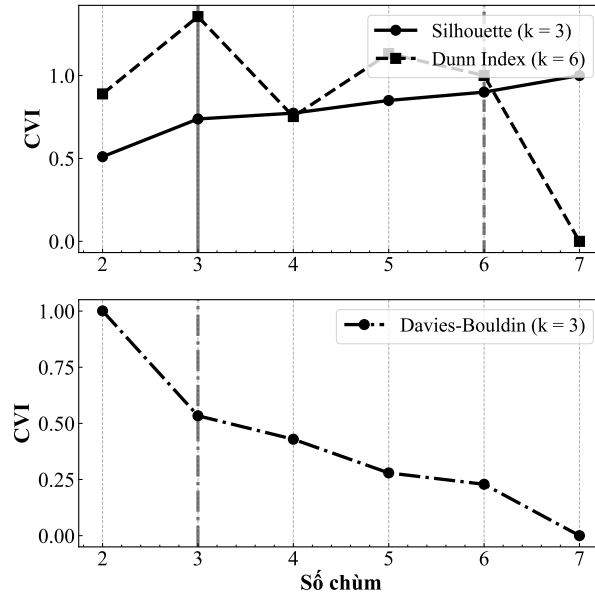
Hình 2.6: Một số chỉ số đánh giá và số chòm tối ưu được đề xuất từ phương pháp khuỷu tay với dữ liệu hàm mật độ ở Ví dụ 1.5
