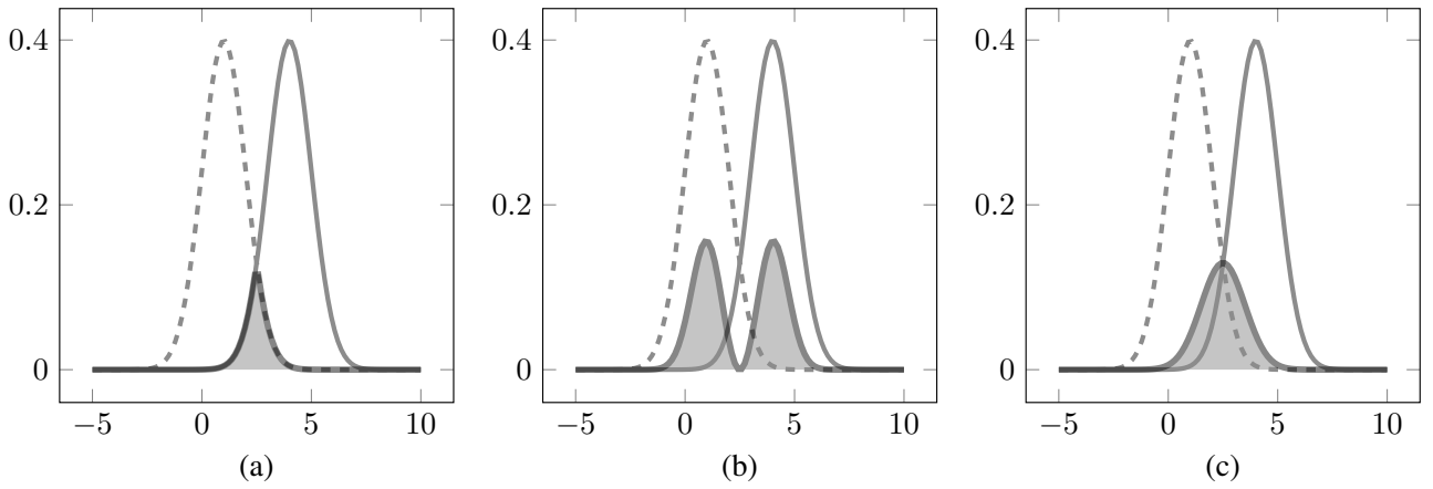
Hình 1.3. Minh họa khoảng cách \mathcal{L}_2 và một vài Affinity phổ biến giữa hai hàm mật độ Gauss \mathcal{N}(1, 1) và \mathcal{N}(4, 1)
