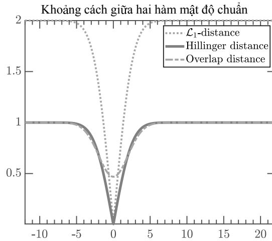
Hình 1.4. Dãy khoảng cách giữa hai hàm mật độ Gauss \mathcal{N}(0, 1) và \mathcal{N}(\mu, 1)
