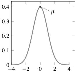
(a) Hàm mật độ Gauss một chiều
