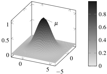
(b) Hàm mật độ Gauss hai chiều
