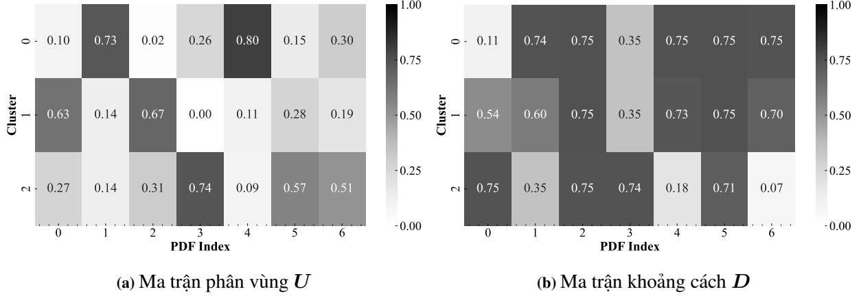
Hình 3.1. Khởi tạo ngẫu nhiên của FCF
