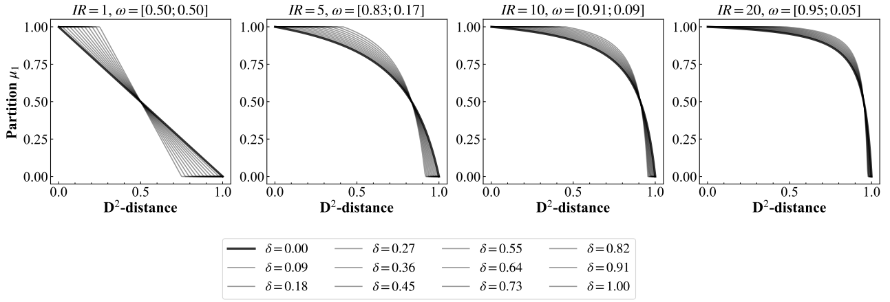
Hình 2.3. Ảnh hưởng của tham số hiệu chỉnh biên \delta trong EM-IFCM qua IR
