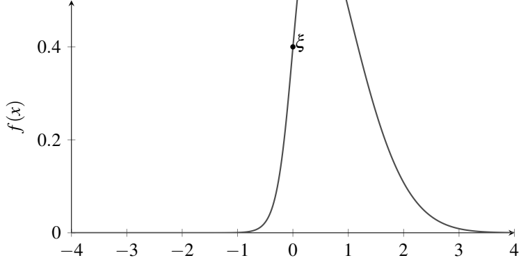
(a) Hàm mật độ Skew-Normal một chiều
