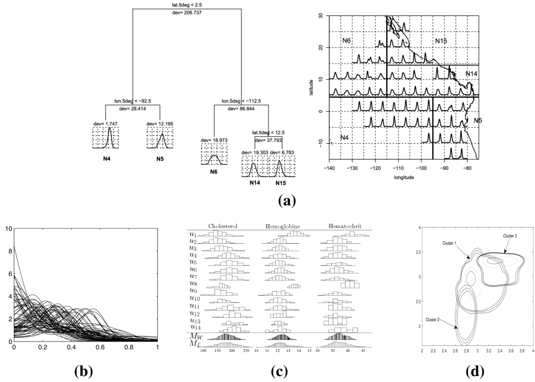
Hình 2.1: Minh họa các dữ liệu hàm mật độ được thu thập trong thực tế từ các nghiên cứu trước đây
