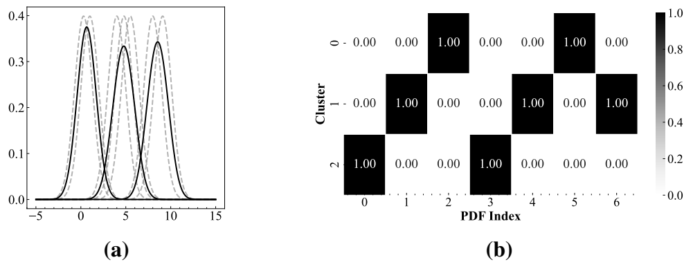
Hình 1.5: Kết quả trọng tâm và ma trận phân vùng của thuật toán KCF đối với Ví dụ 1.4 Chú thích: Hình (a) trọng tâm cụm bằng nét liền và dữ liệu hàm mật độ nét đứt, và (b) ma trận phân vùng cứng của KCF. Nguồn: Minh họa của tác giả.
