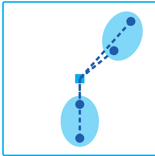
(e) Liên kết Ward
