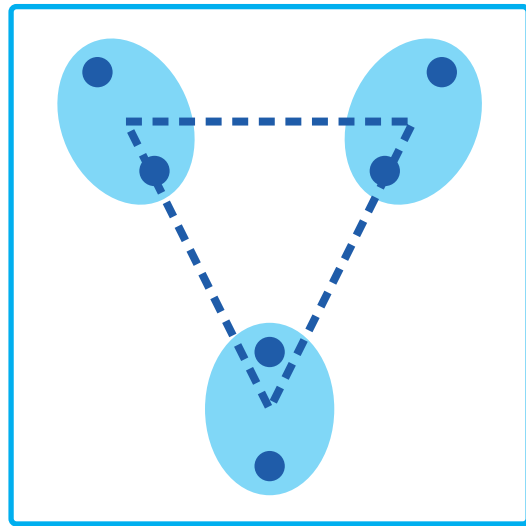
(c) Liên kết tâm (UPGMC)
