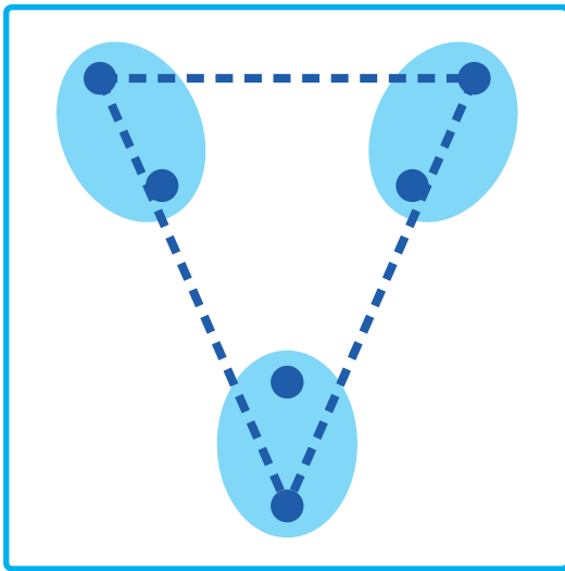
(b) Liên kết đủ (CLINK)
