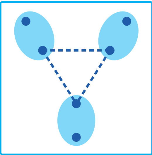
(a) Liên kết đơn (SLINK)
