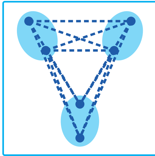
(d) Liên kết trung bình (UPGMA)
