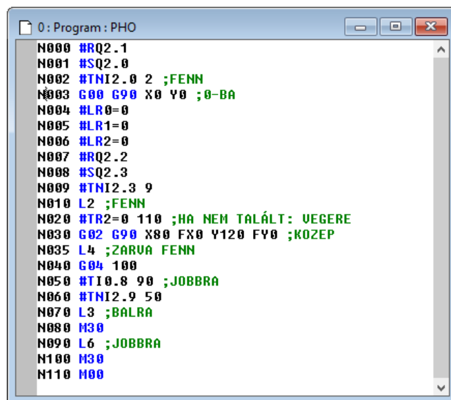
Ábra 4: Főprogram
