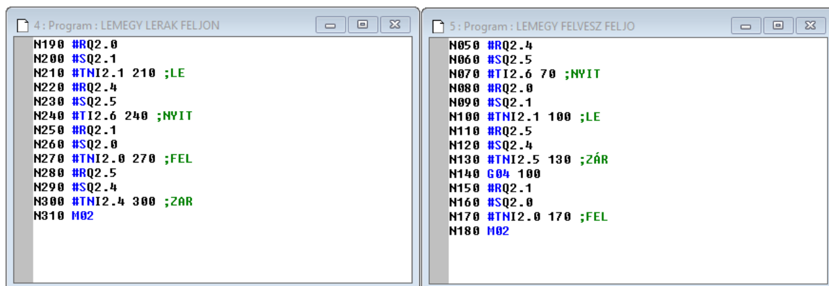
Ábra 3: Segédprogramok
