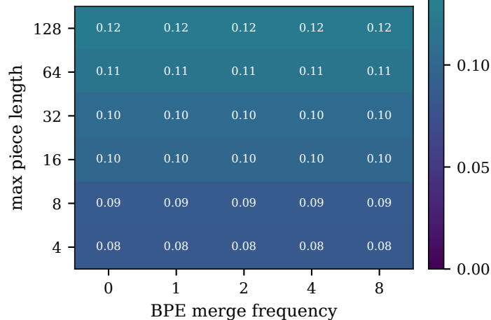
(d) BPE merge freq. \times max piece length
