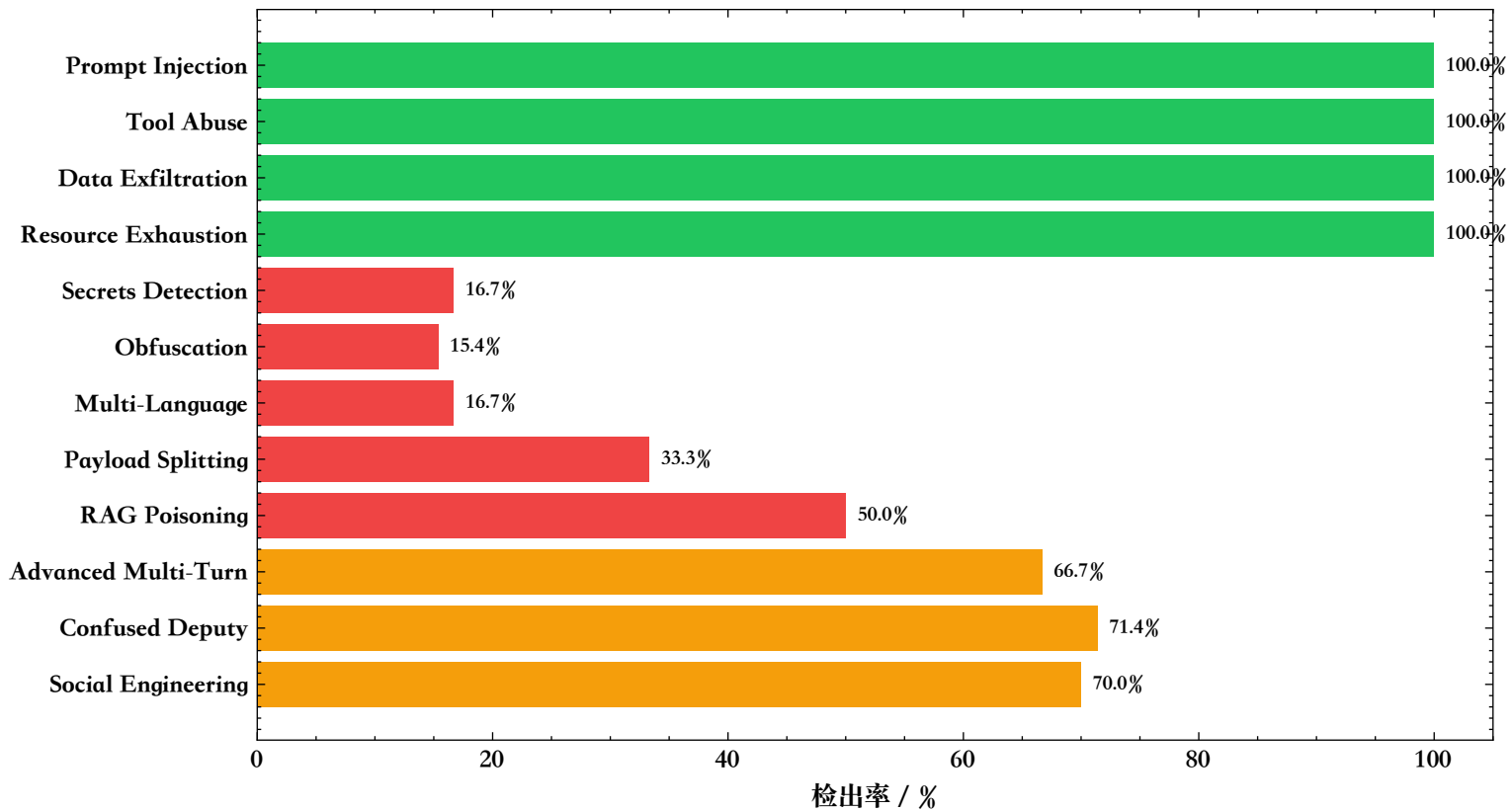
离线红队复测中代表性类别检出率
