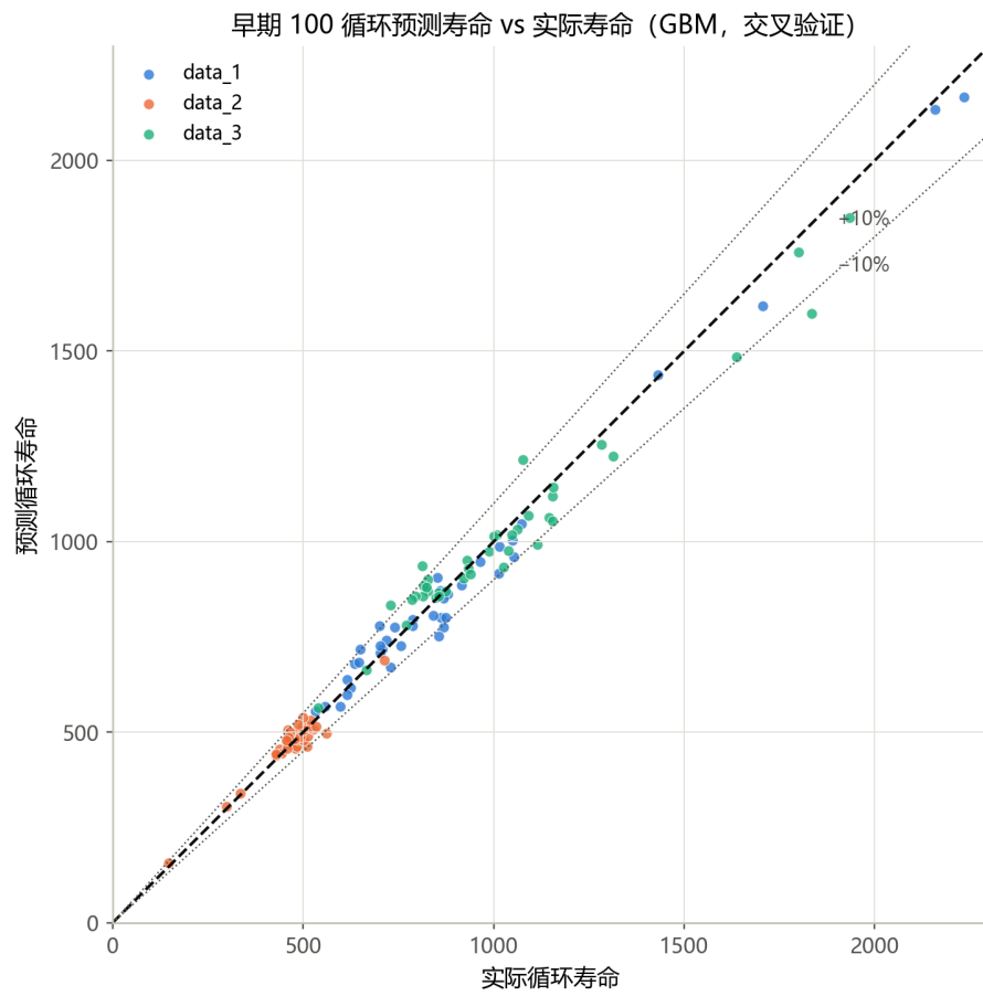
图 12 早期 100 循环预测寿命 vs 实际寿命 (GBM, 交叉验证)
