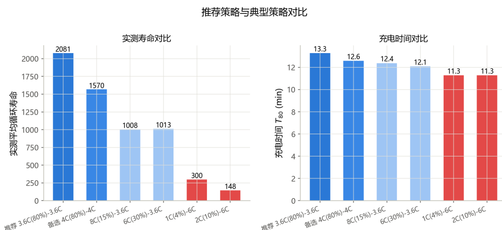
图 18 推荐策略与典型策略的实测寿命与充电时间对比
