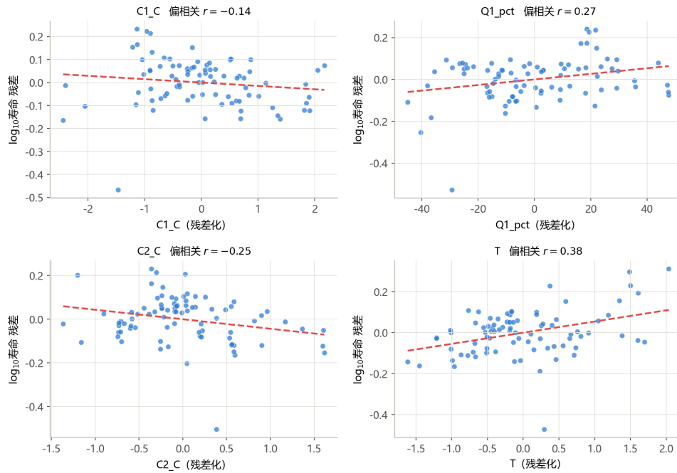
图 8 偏回归图 (控制其他变量与批次后, 各参数与寿命的关系)
