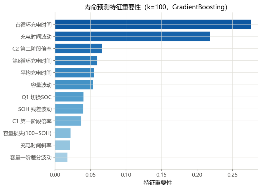
图 13 寿命预测特征重要性 ( k = 100 , GBM)
