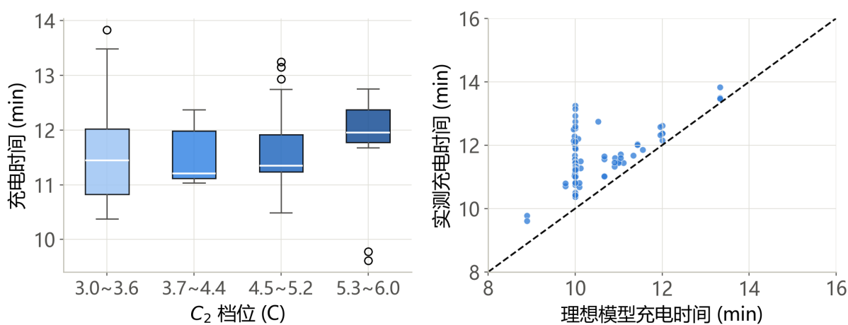
图 6 充电时间分析：随 C_2 档位分布与理想模型对比 (standard, n=84)
