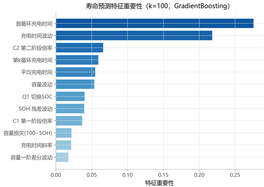
图 15 寿命预测特征重要性 ( k = 100 , GBM)
