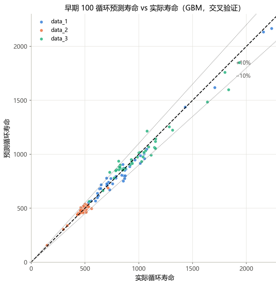
图 14 早期 100 循环预测寿命 vs 实际寿命 (GBM, 交叉验证)
