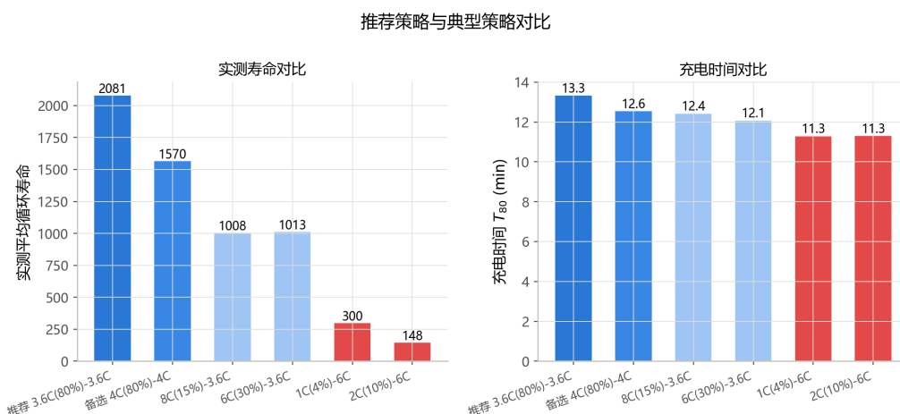
图 20 推荐策略与典型策略的实测寿命与充电时间对比
