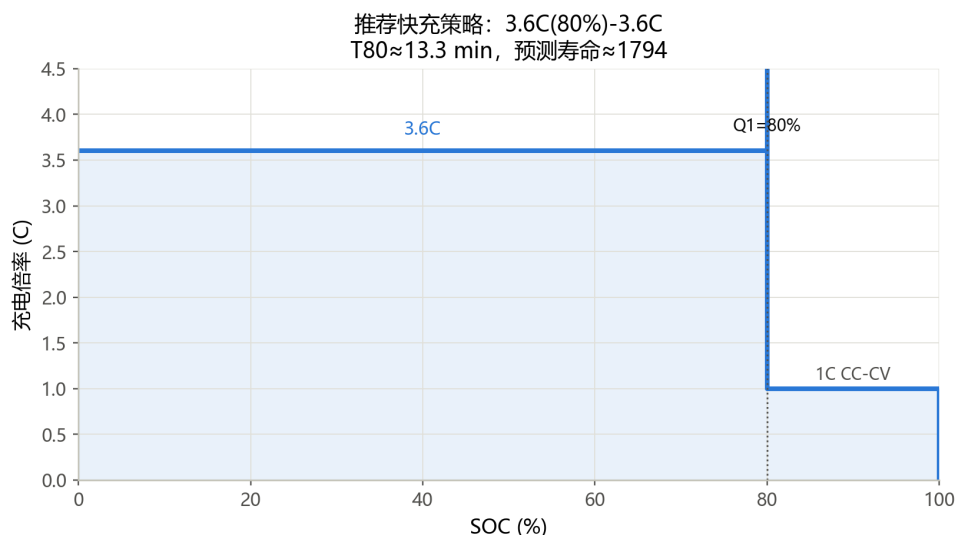
图 19 推荐快充策略电流剖面 (3.6C(80%)-3.6C)
